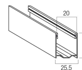
Guida in alluminio A27 GUAL..27M 25,5 x 30 mm
